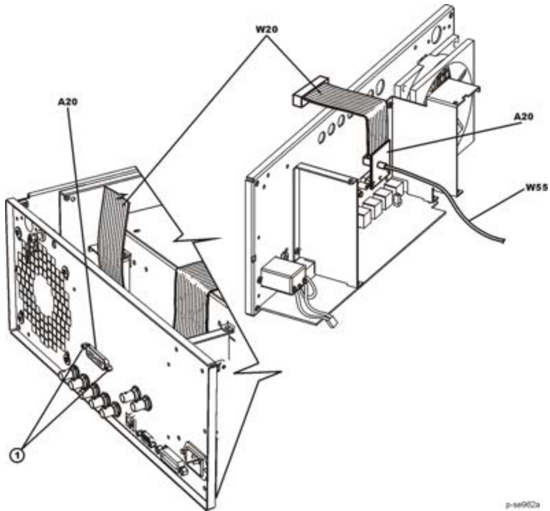
Figure 3-27 A20 SMI
